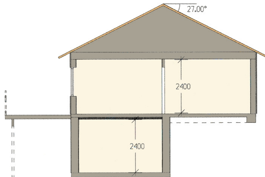
Sektion A-A
